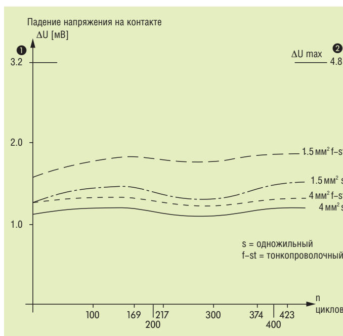
Испытания при длительном циклическом нагреве, серии 281 (4 мм 2 , 35 А). На диаграмме учтены изменения напряжения источника питания..
