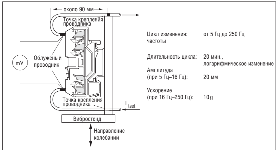
Рис. II: Установка
